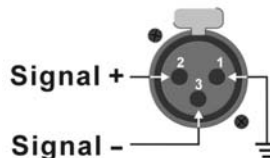
Abb. 4 Eingangsbuchse
