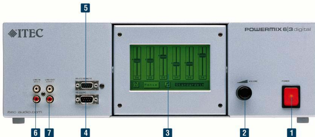
Abb. 1 POWERMIX Frontansicht
