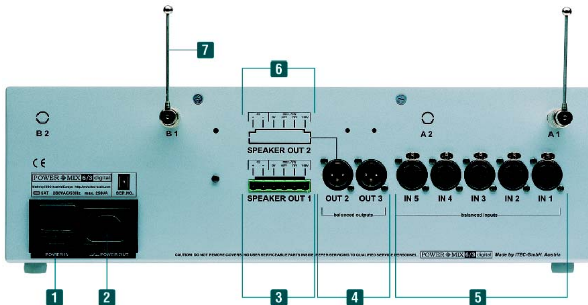
Abb. 2 POWERMIX Rückansicht
