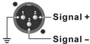
Abb. 3 Ausgangsbuchse
